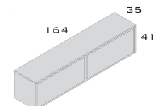
GE-47 SZAFKA WISZĄCA
